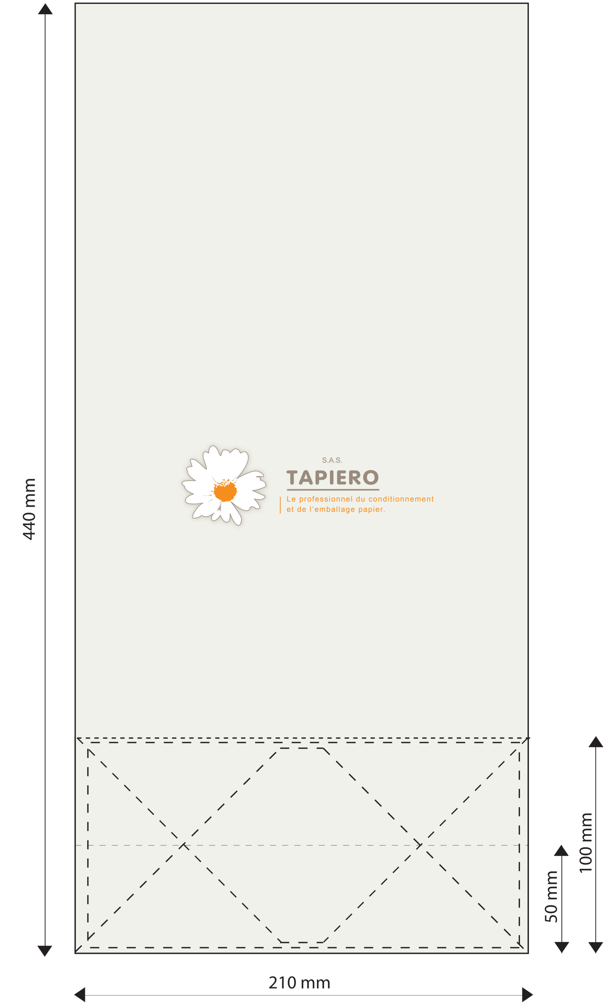
Sac plié : Vue recto
